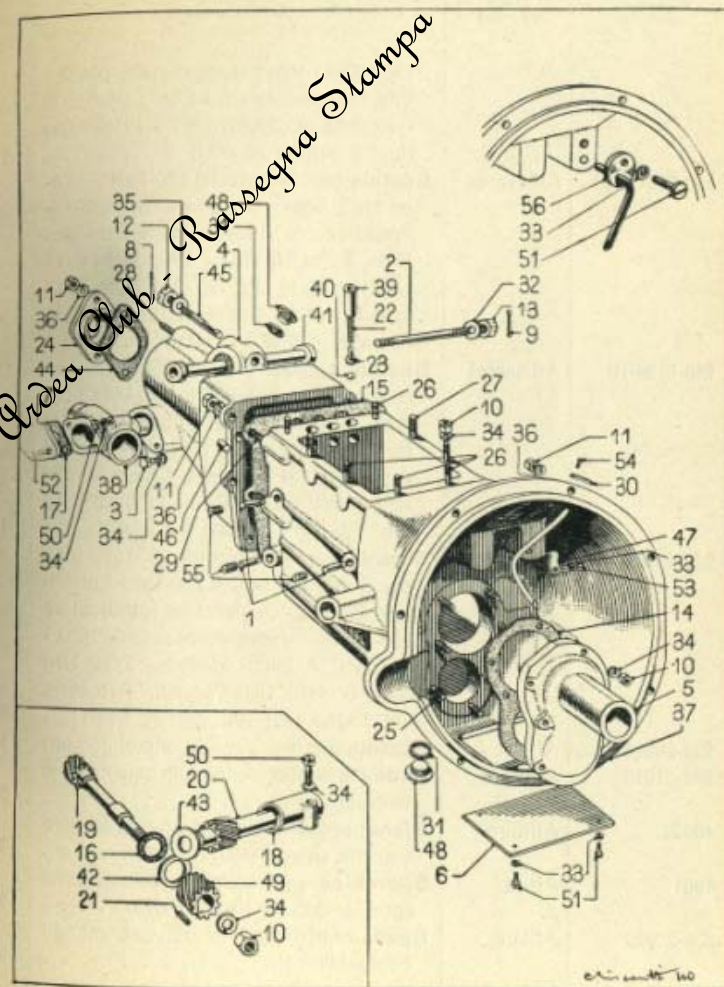
TAV. 22. SCATOLA CAMBIO VELOCITÀ - COMANDO CONTACHILOMETRI
