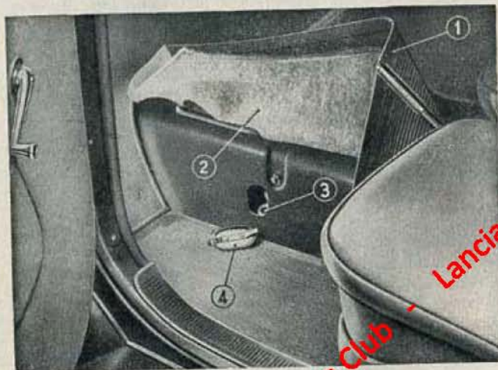
Fig. 24. - - Lubrificazione del cambio di velocità.
