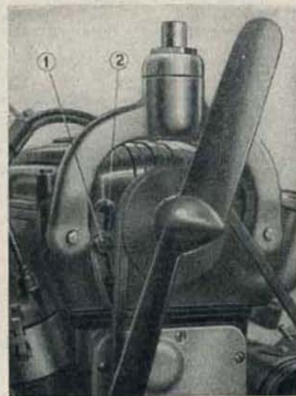
Fig. 21. - Regolazione della tensione della cinghia del ventilatore.
