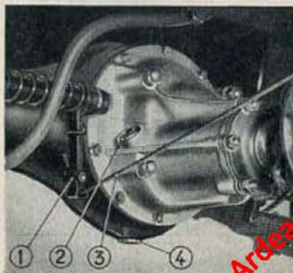
Fig. 27. Gruppo differenziale e organi vari.
