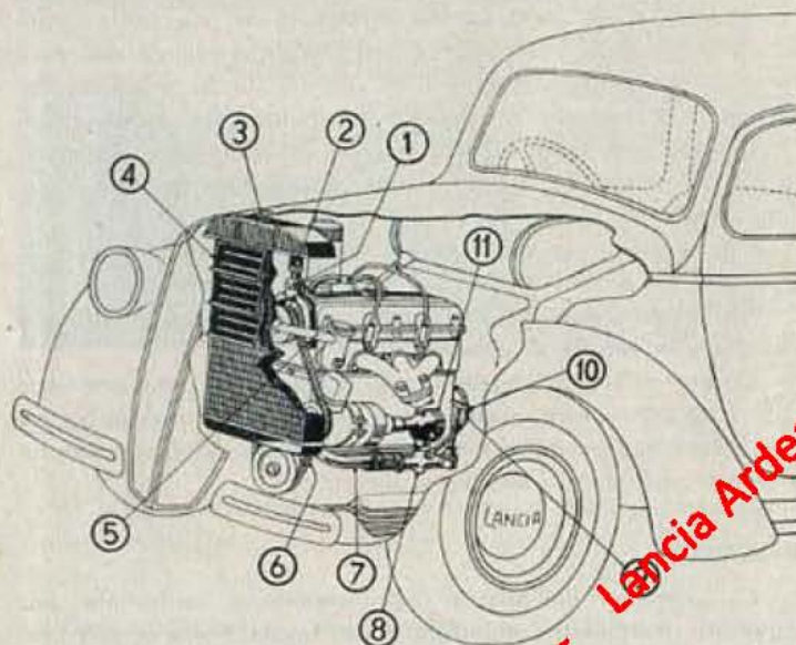
Fig. 18. - Schema raffreddamento motore.
