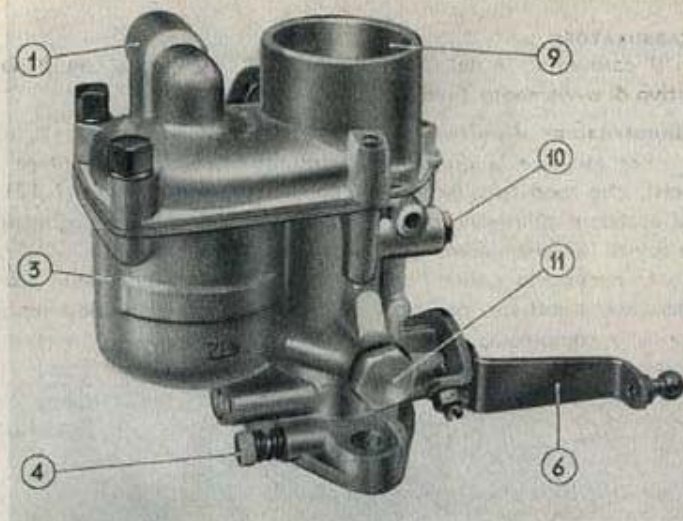
Fig. 12. - Vista esterna carburatore.
