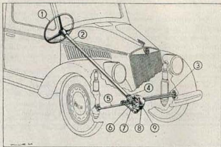
Fig. 29. - Schema dello sterzo.
