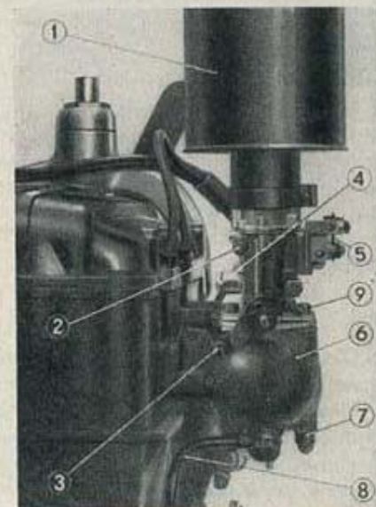
Fig. 13. - Carburatore montato sul motore.
